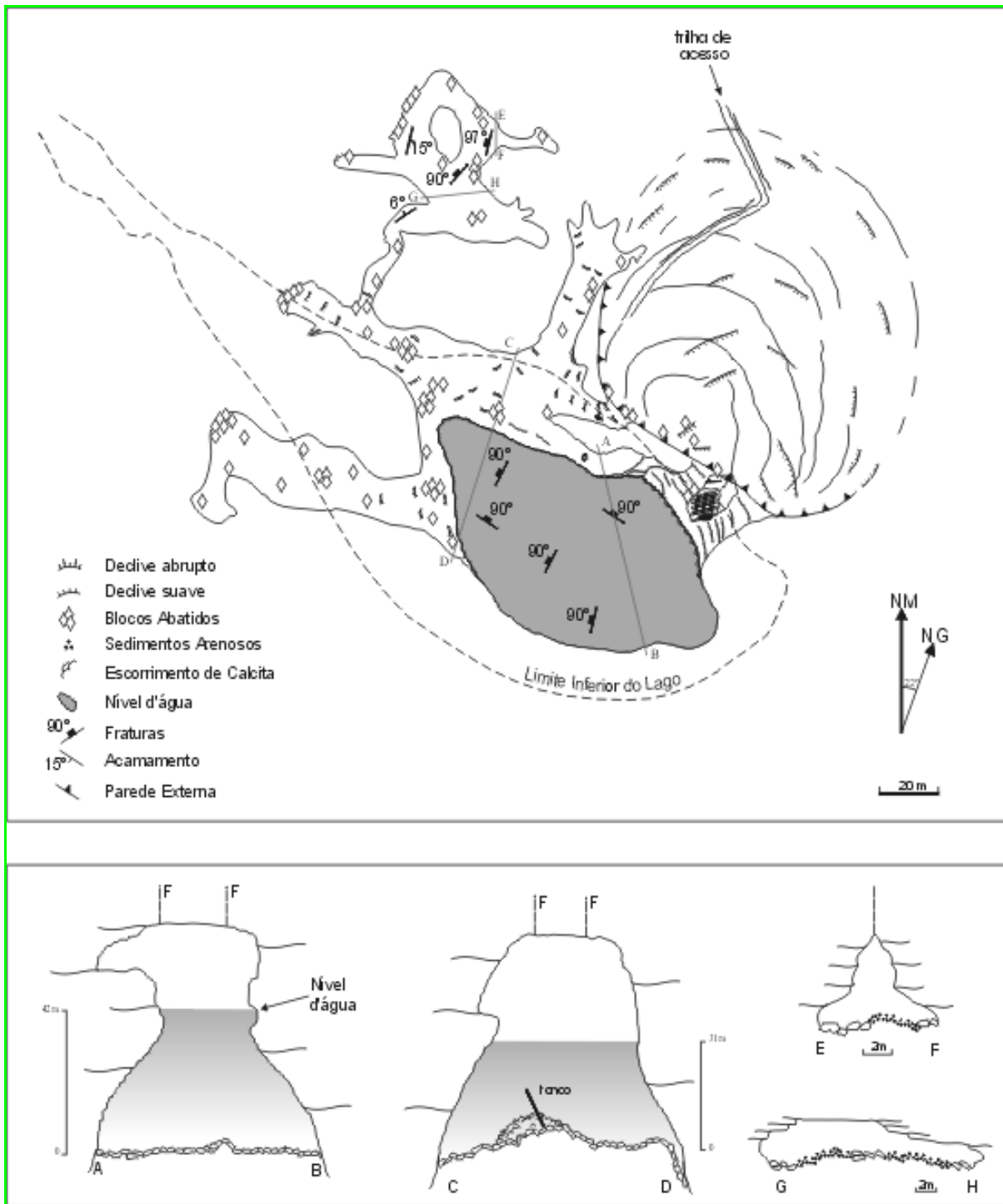
Figura 3 - Mapa planimétrico e seções transversais da caverna Poço Encantado. Base topográfica adaptada do Grupo Bambuí de Pesquisas Espeleológicas.
