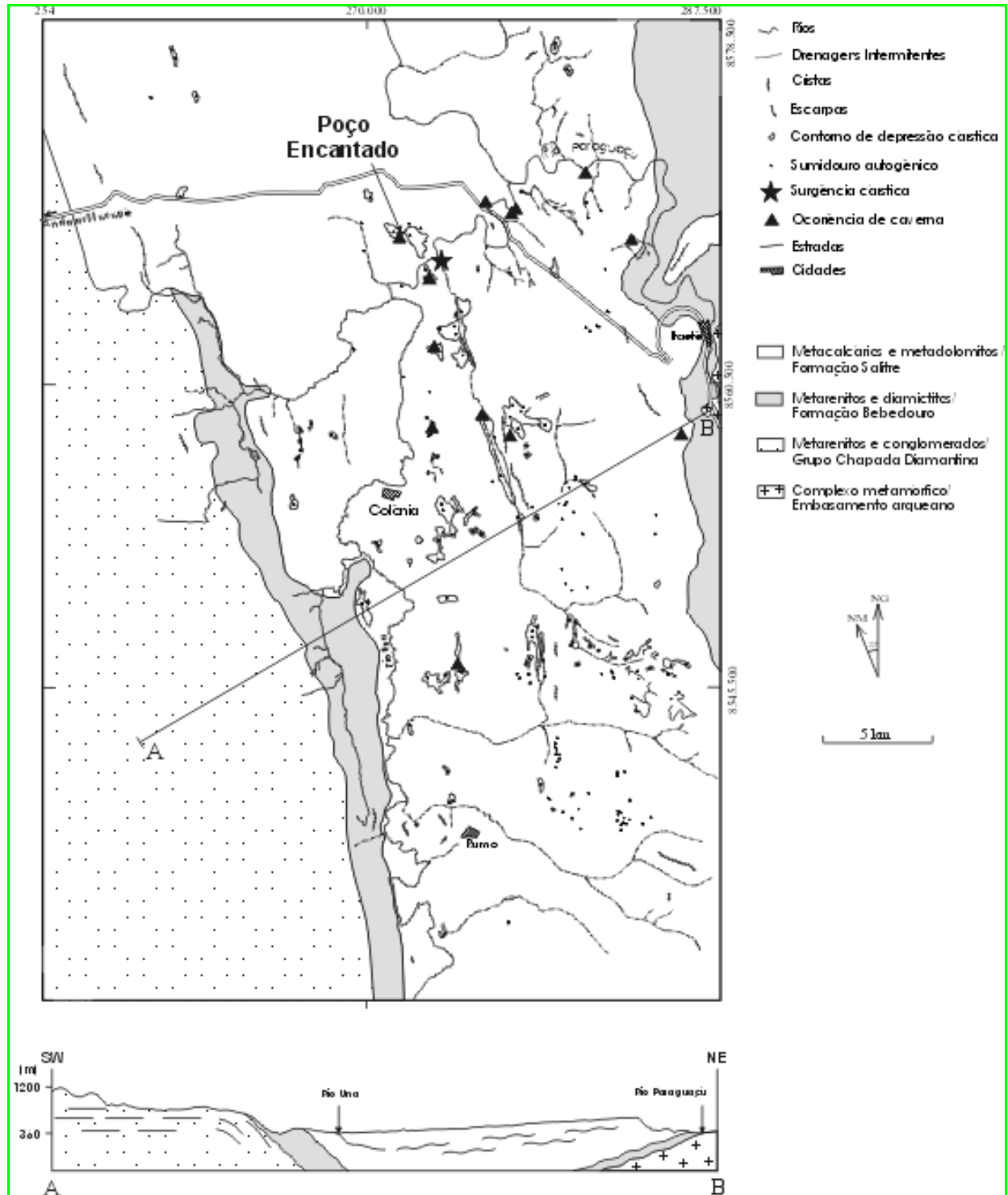
Figura 2 - Situação geológica da caverna Poço Encantado e aspectos morfológicos do carste da bacia do rio Una. Adaptado de Pereira (1998).
